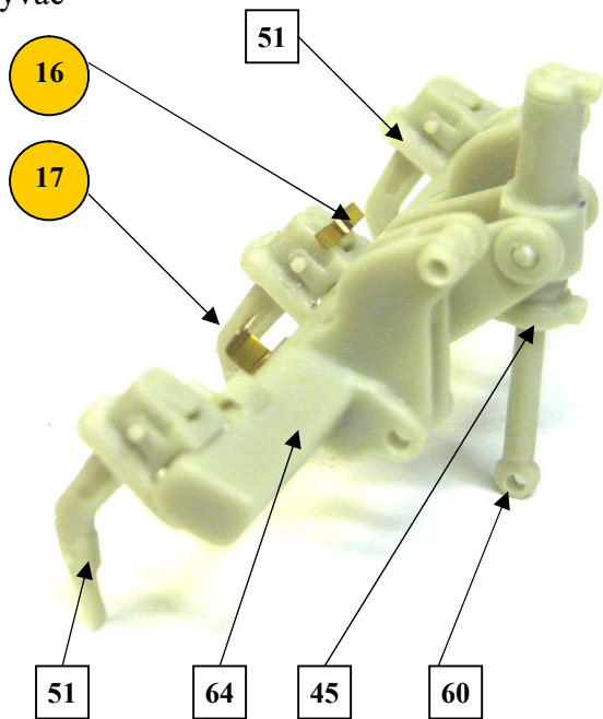
Multi-Shank Riepper Rozrývač
